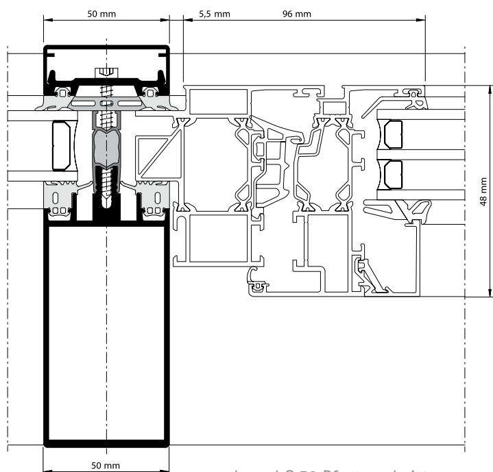
heroal C 50 Pfostenschnitt-darstellung mit Einselelement
